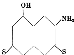
R R Säure.
